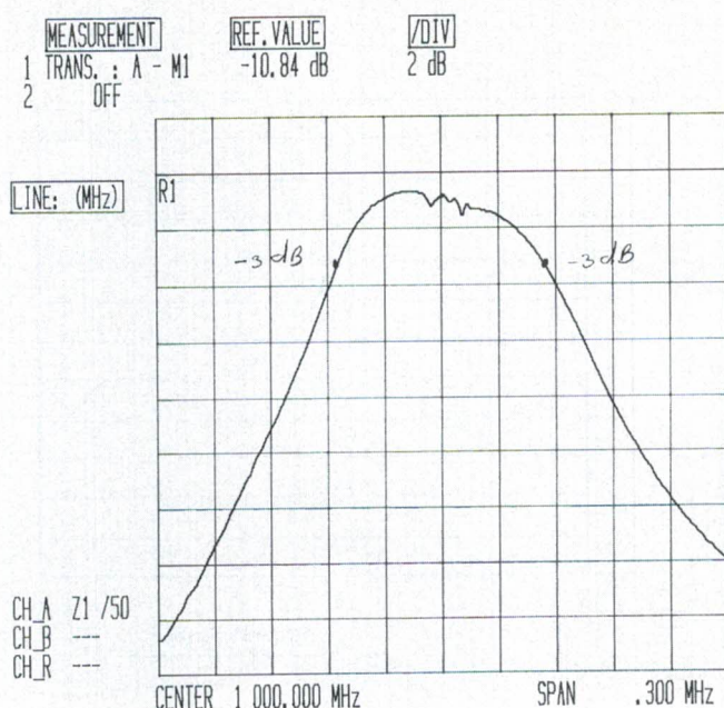
Afb. 5 Statische selectiviteit MF filters gemeten na 2e MF.
