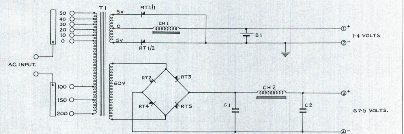
Circuit diagram voor 301 power pack.
